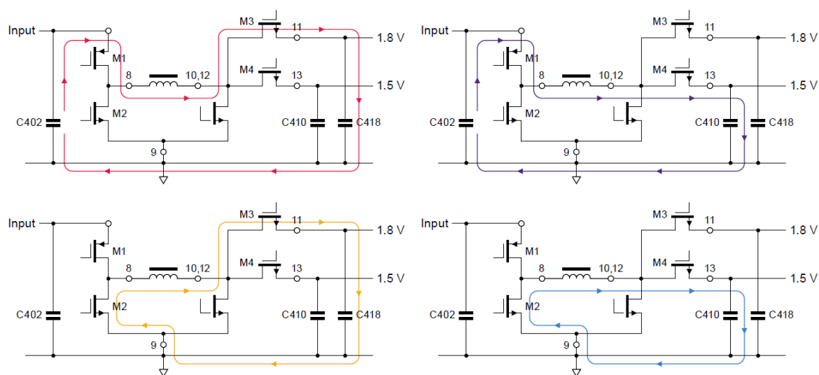
图 11.降压模式下 DC-DC 转换器的两路输出的电流环路
