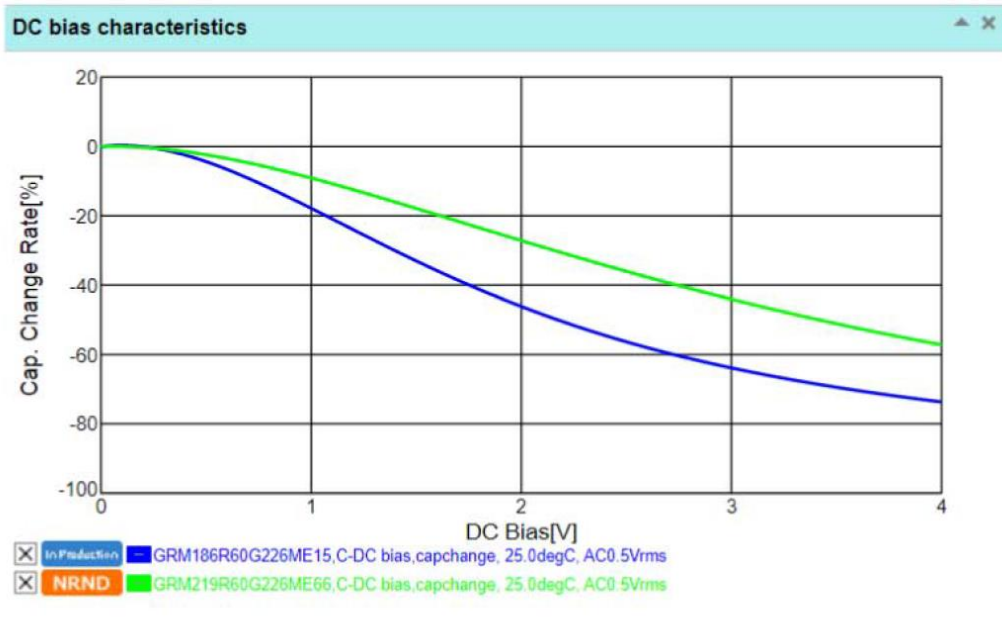
图 15. 电容变化与直流偏置电压的关系
