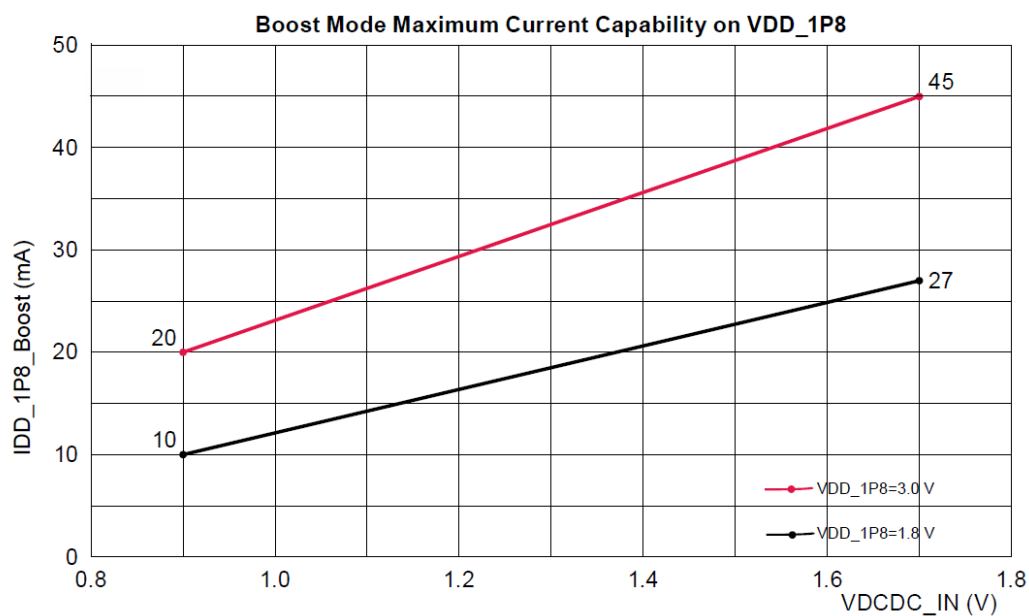
图 18.最大 IDD_1P8_boost 与 VDCDC_IN 输入电压的关系
