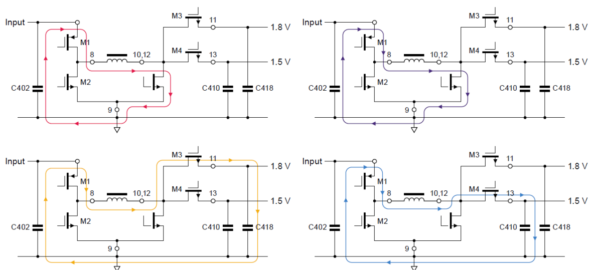
图 12.升压模式下 DC-DC 转换器的两路输出的电流环路
